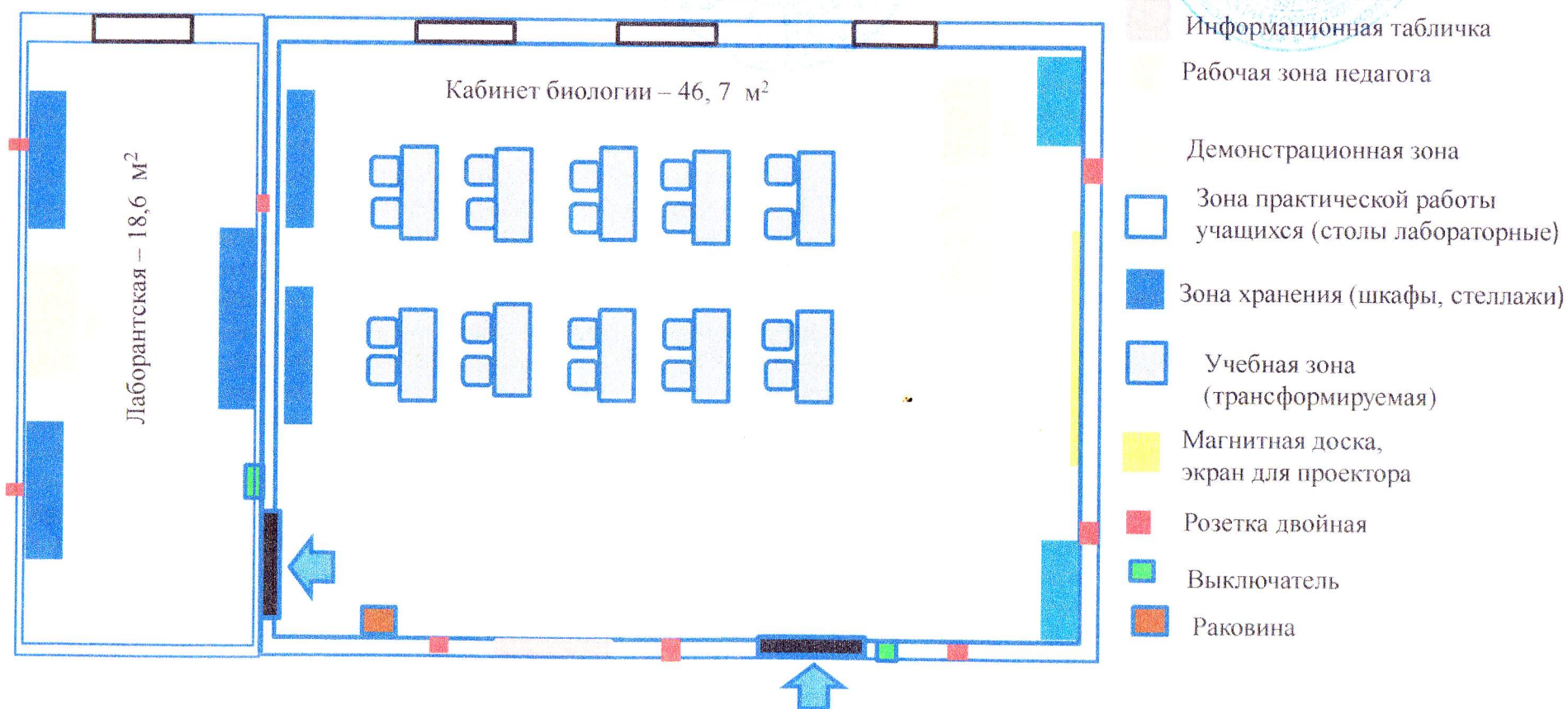
План –схема биологической лаборатории (с лаборантской) Центр «Точка роста» на базе ГБОУ СОШ с. Колывань (65,3 м 2 )
